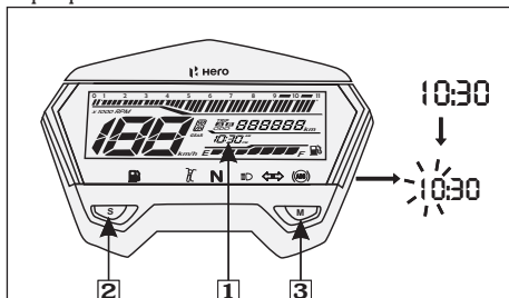
(1) Reloj digital
