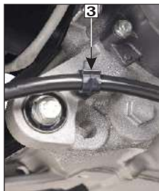
(3) Guía del cable del freno trasero (4) Tapa del filtro del aceite
