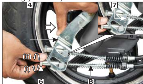
(6) Segunda tuerca de ajuste (i) Disminuir el juego libre (ii) Aumentar el juego libre
